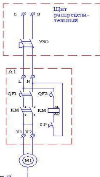
Эл.схема 2
