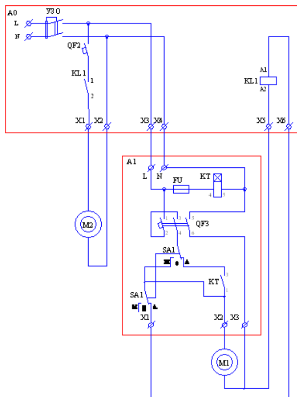
Эл.схема 1
