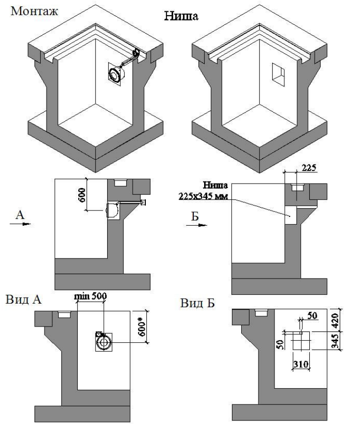
Рисунок 4 (Установка в переливной бассейн)
