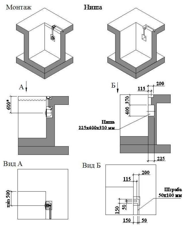
Рисунок 4 (Установка в переливной бассейн)
