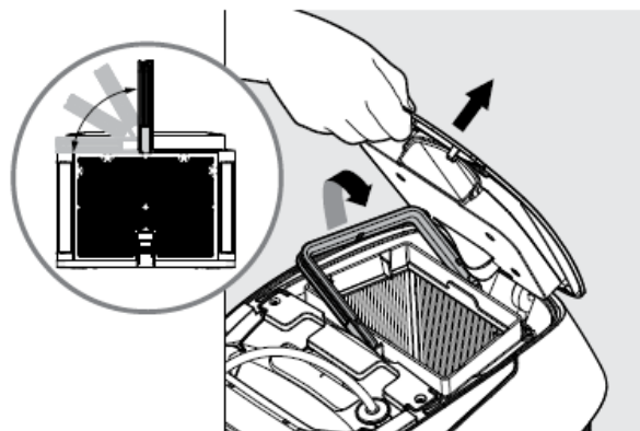
6.1.2 При открытии крышки фильтра, ручка автоматически поднимается.
