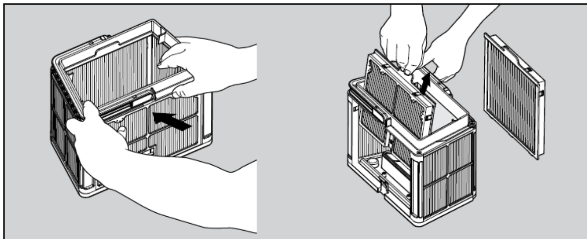
6.2.1 Снимите стенки с помощью больших пальцев.
