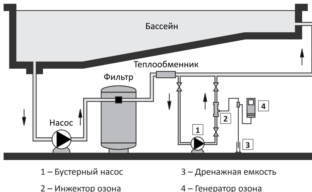
Установка озонатора Triogen T2 без системы дегазации
