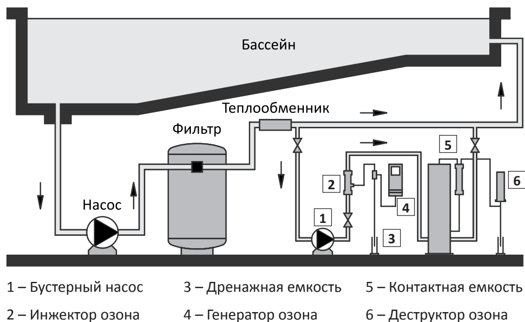
Установка озонатора Triogen T2 с системой дегазации
