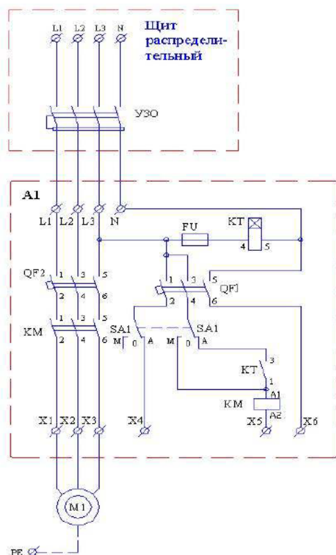
Эл.схема 1
