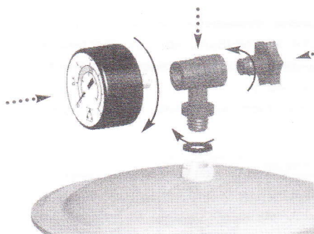
монтаж манометра при боковом вентиле
