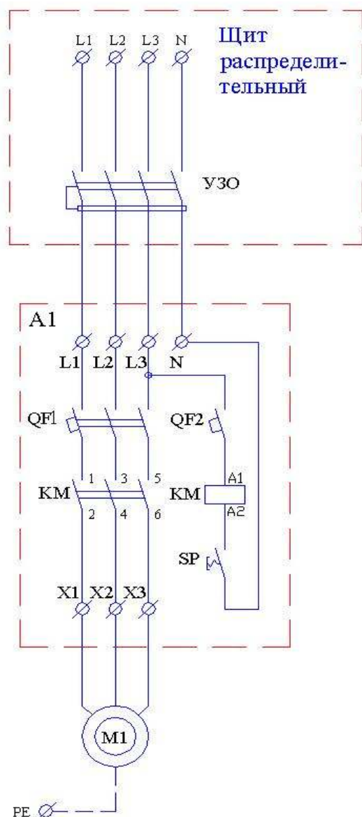
Эл.схема 2
