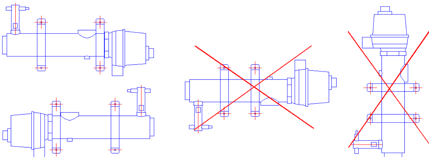
штатное положение
