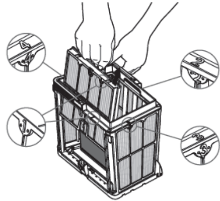
6.2.3 Снимите оставшиеся стенки по их нумерованному порядку их: 2 → 3 → 4.
