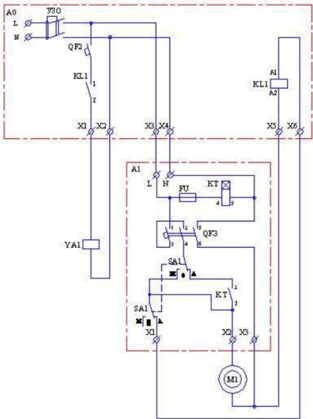
Эл.схема 1 Таблица условных обозначений для
