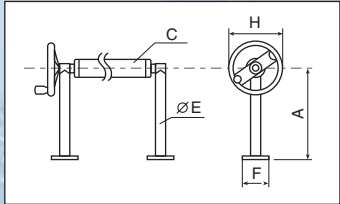
Телескопическое устройство намотки неподвижное
