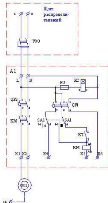
Эл.схема 1
